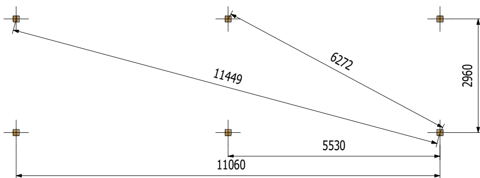
A-A ( 1 : 100 )
